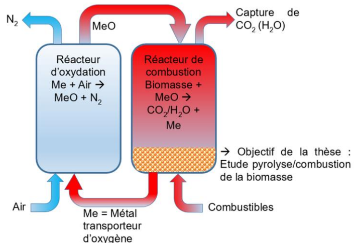
Figure 1 : Schéma de la technologie CLC
